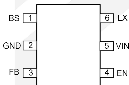
SOT23-6
