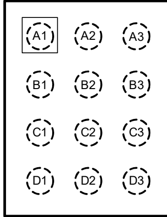
WLCSP-12 Pins
